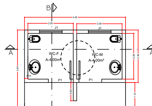
PLANTA BAIXA ESC-1/100
