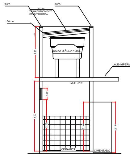
CORTE-BB ESC-1/100
