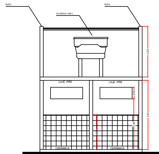
CORTE-AA ESC-1/100
