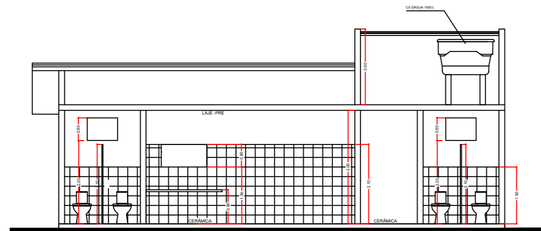
CORTE-AA ESC-1/100
