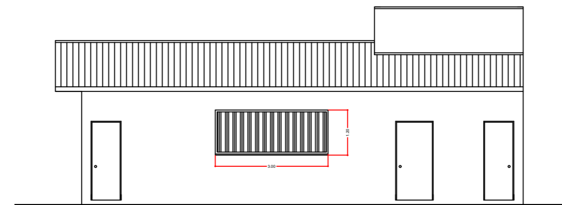
FACHADA ESC-1/100
