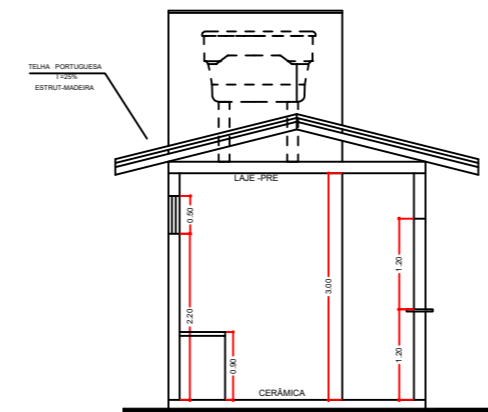
CORTE-BB ESC-1/100
