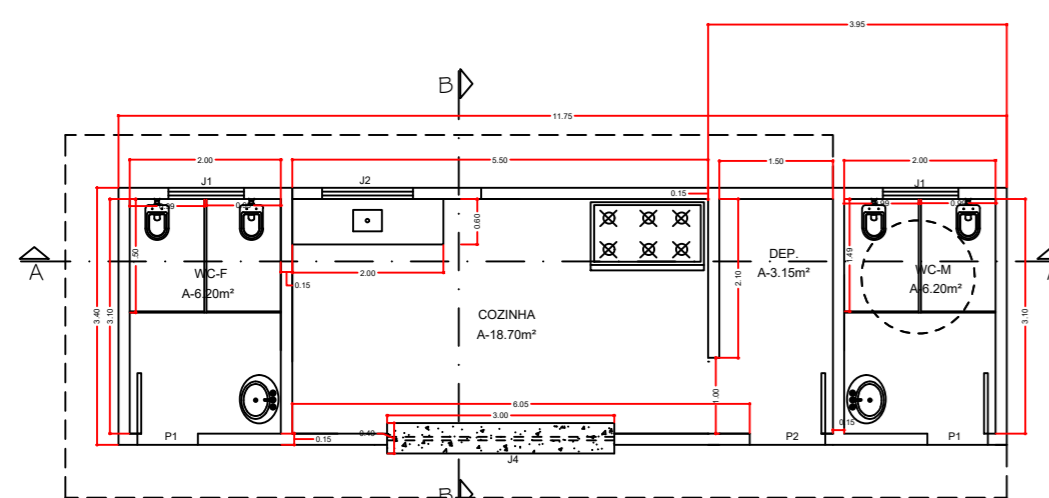
PLANTA BAIXA ESC-1/100 A.40.00m²
