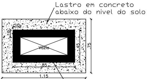
Planta ESCALA 1/25
