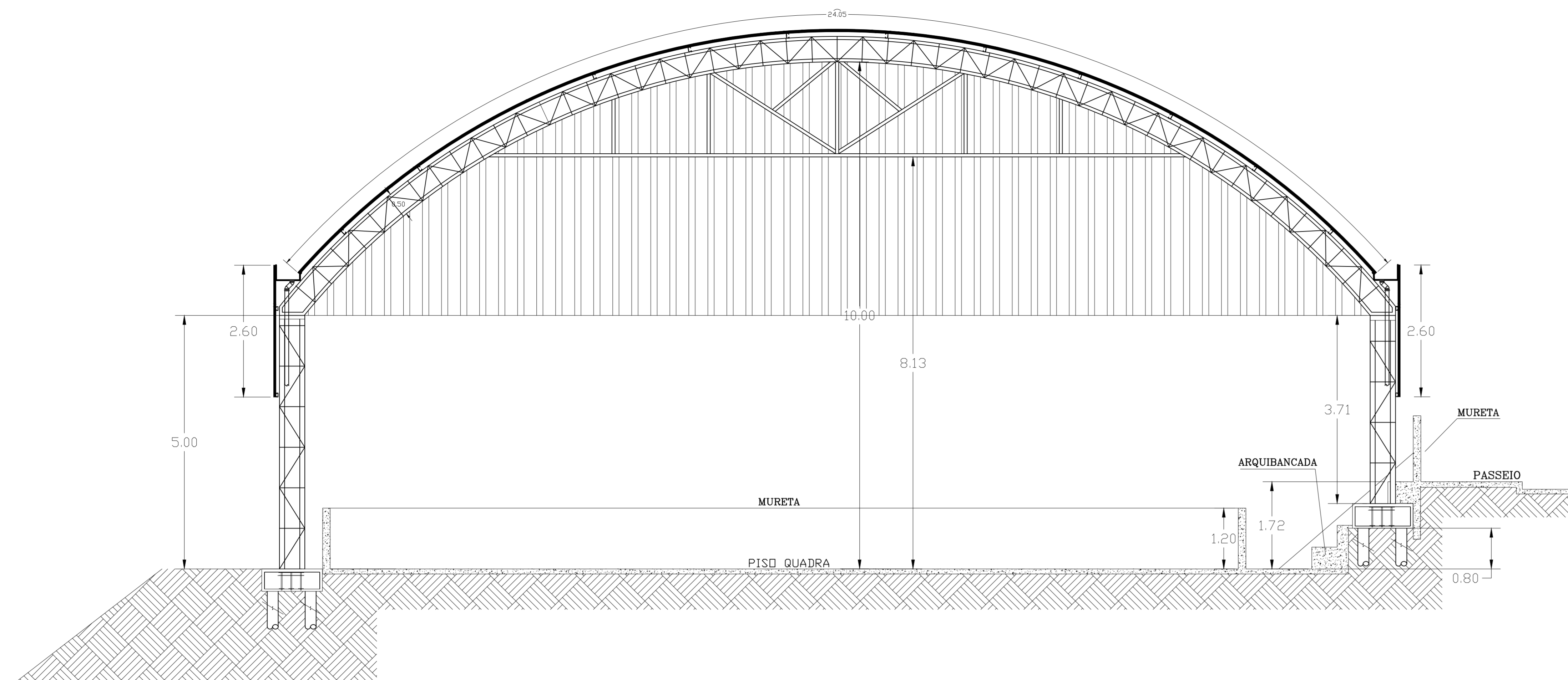
VISTA - BB ESC. 1: 100
