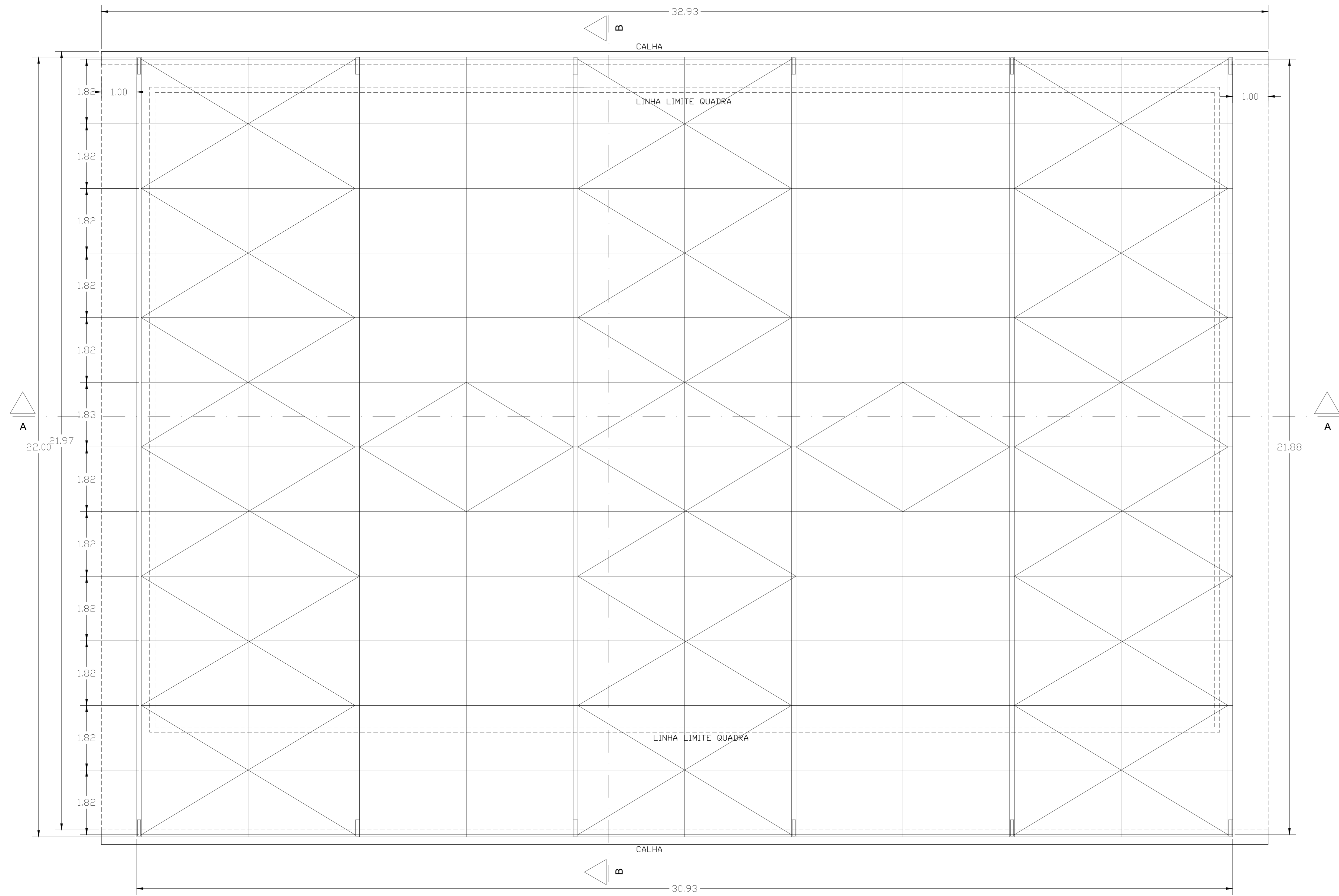
PLANTA COBERTURA Escala: 1/50
